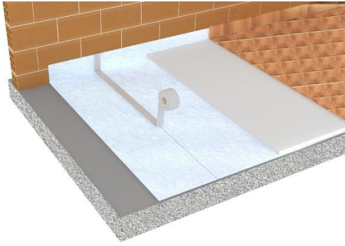
Figura 7.5: Instalación de AISREC REFLEX PRIME 308EB sobre el paramento horizontal.
