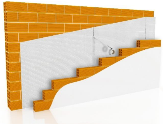
Figura 7.4: Instalación en vertical con fijación sobre paramento continuo.
