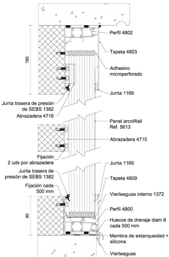
Figura 5.15: Instalación vertical para sistemas con grandes dilataciones.
