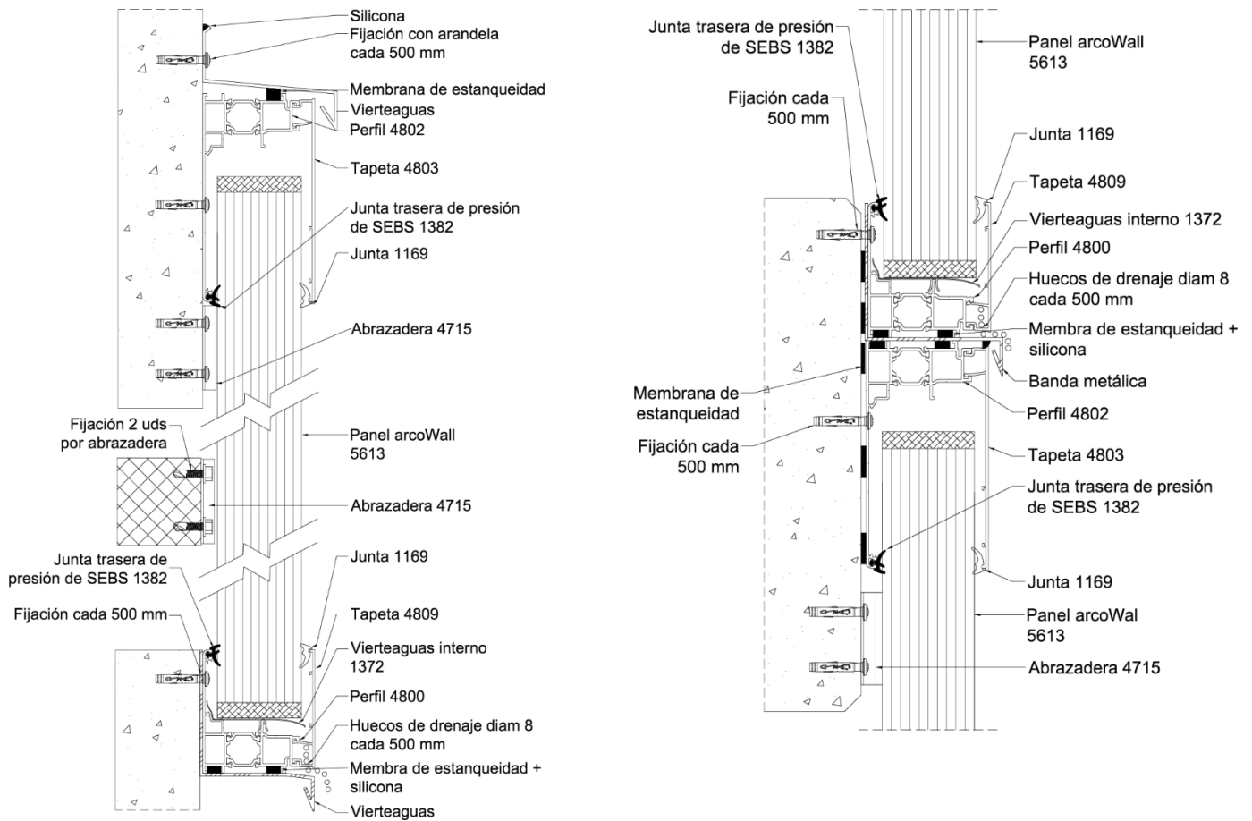
Figura 5.17: Instalación vertical para sistemas con grandes dilataciones y acabado con vierendeaguas.
