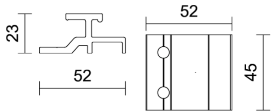
Figura 2.6b: Abrazadera 4716.
