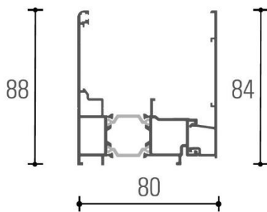
Figura 2.5a: Perfil 4800 + tapeta 4809.
