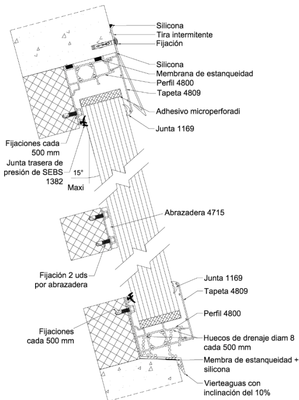
Figura 5.11: Instalación inclinada para sistemas con pequeñas dilataciones.
