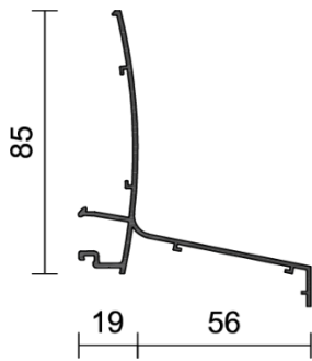
Figura 2.4c: Tapeta 4807 de aluminio base curva con vierteaguas.
