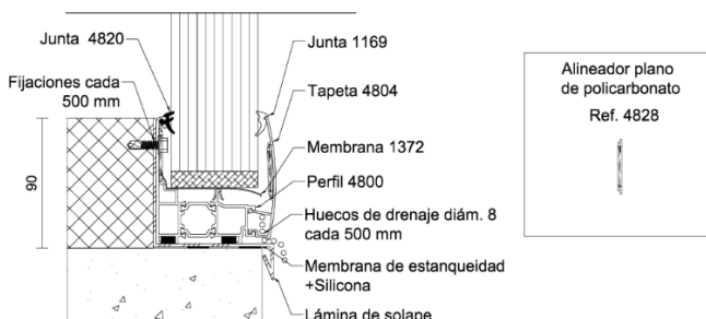
Figura 5.5: Arranque del sistema con perfil 4800 y tapeta 4804.
