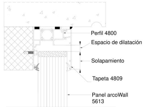
Figura 5.2: Coronación del sistema con perfil 4800.
