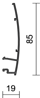
Figura 2.4a: Tapeta 4804 de aluminio base-lateral-superior curva.
