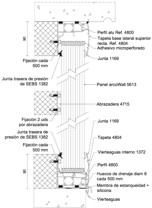
Figura 5.19: Instalación vertical para sistemas con pequeñas dilataciones con tapetas curvadas sin vierteaguas interno 1372.
