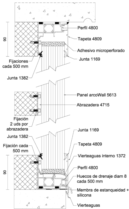
Figura 5.9: Instalación vertical para sistemas con pequeñas dilataciones.
