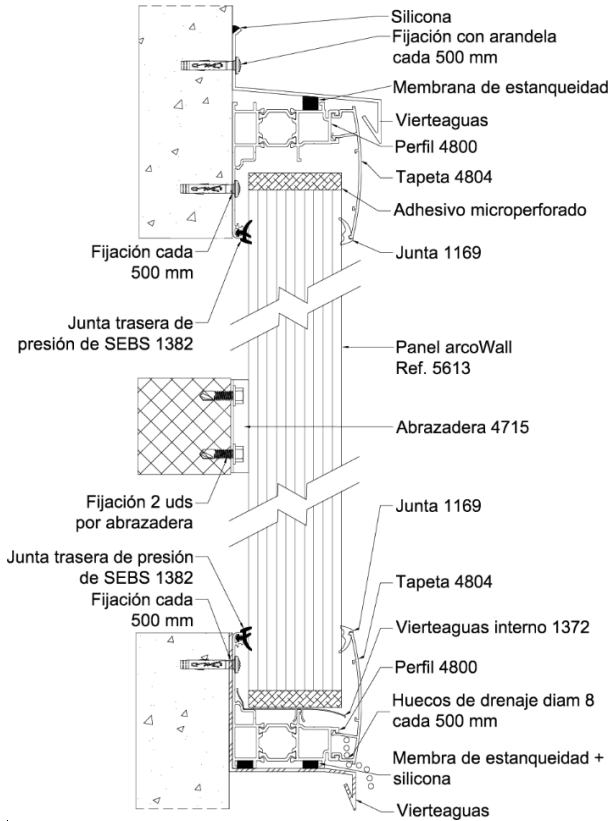
Figura 5.21: Instalación vertical para sistemas con pequeñas dilataciones con tapetas curvadas con vierteaguas superior y sin vierteaguas interno 1372.
