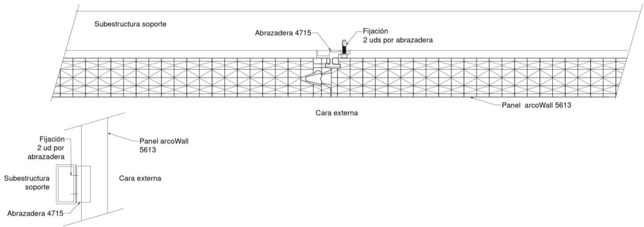
Figura 5.7: Instalación de las abrazaderas en el largo del sistema.
