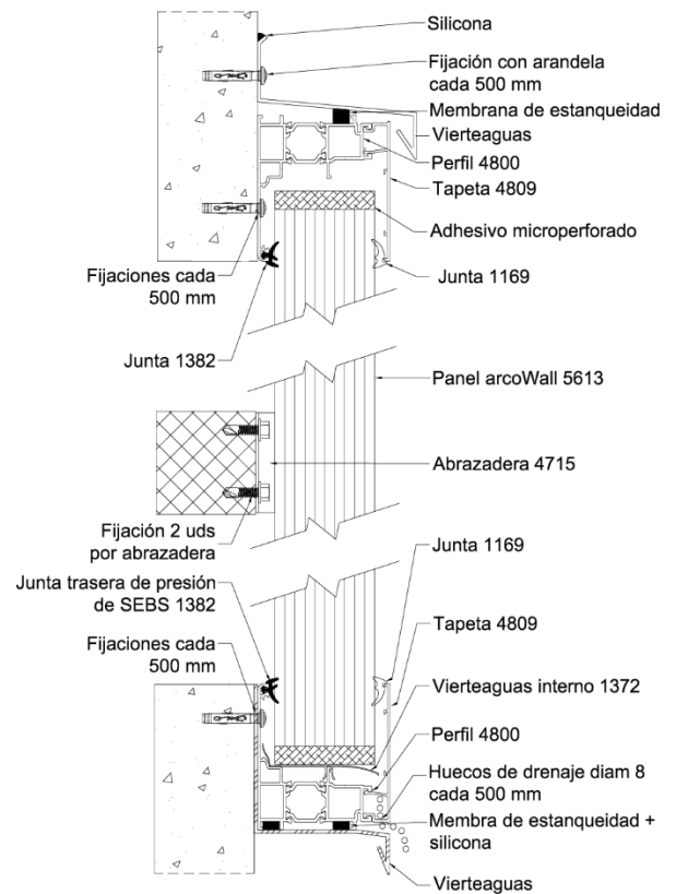
Figura 5.10: Instalación vertical para sistemas con pequeñas dilataciones y acabado superior con vieriteaguas.
