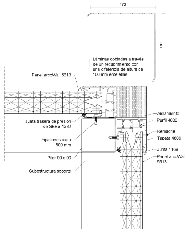
Figura 5.14: Instalación en esquina con perfiles rectos.
