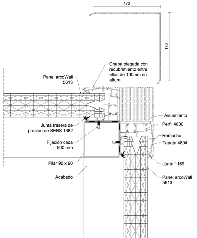
Figura 5.24: Instalación en esquina con perfiles curvados.
