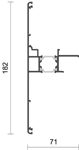
Figura 2.3c: Perfil 4805.
