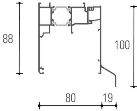
Figura 2.5c: Perfil 4800 + tapeta 4819.
