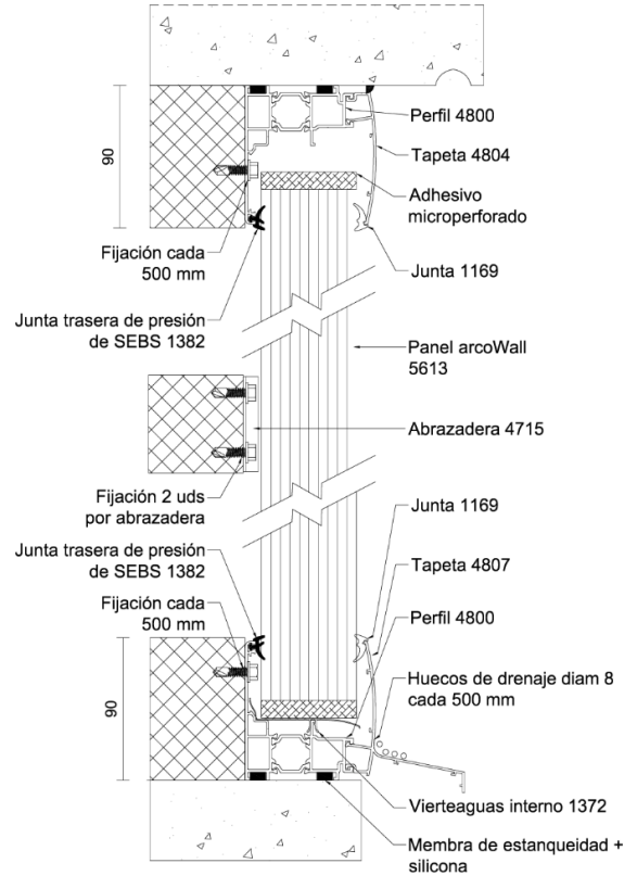
Figura 5.20: Instalación vertical para sistemas con pequeñas dilataciones con tapetas curvadas con vierteaguas interno 1372.
