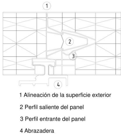
Figura 5.1: Detalle del encastre entre paneles.
