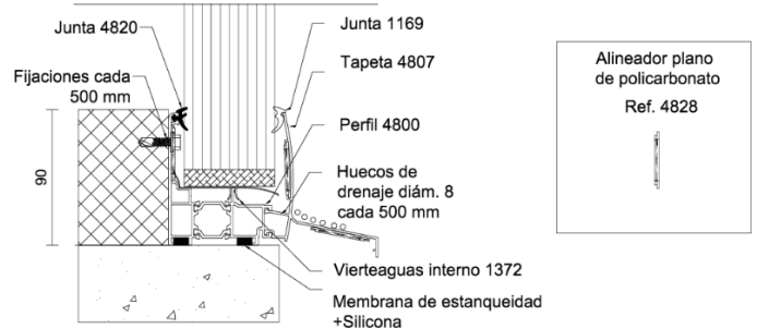
Figura 5.6: Arranque del sistema con perfil 4800 y tapeta 4807.
