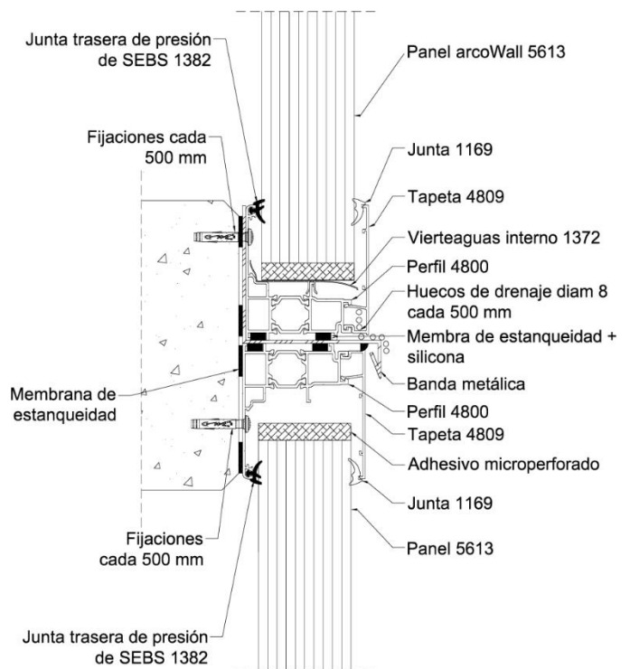
Figura 5.12: Unión de dos paneles con pequeñas dilataciones - con dos perfiles 4800.
