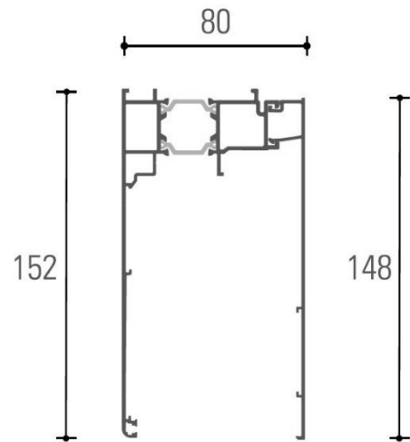
Figura 2.5d: Perfil 4802 + tapeta 4803.
