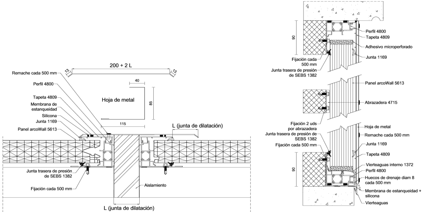
Figura 5.16: Junta de dilatación entre paneles con perfiles rectos.
