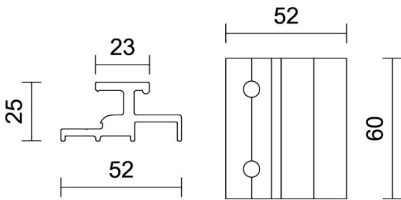
Figura 2.5e: Perfil 4805 + tapeta 4808.
