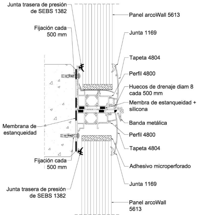
Figura 5.23: Unión de dos paneles con pequeñas dilataciones y perfiles curvados – con dos perfiles 4800.
