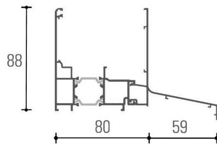
Figura 2.5b: Perfil 4800 + tapeta 4831.
