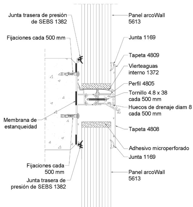
Figura 5.13: Unión de dos paneles con grandes dilataciones - con perfil 4805 y tapeta 4808.
