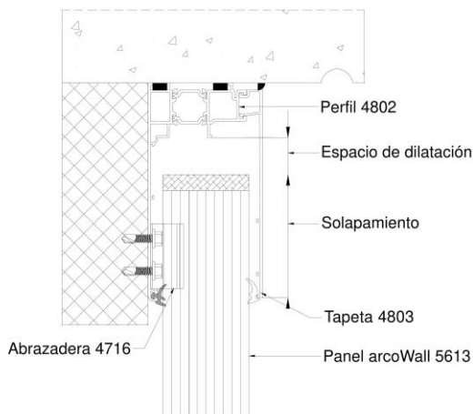
Figura 5.3: Coronación del sistema con perfil 4802.
