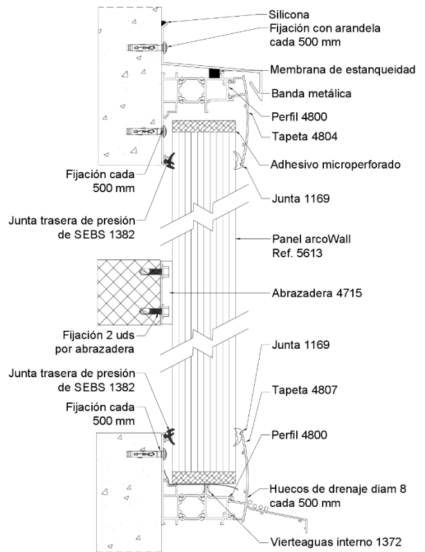
Figura 5.22: Instalación vertical para sistemas con pequeñas dilataciones con tapetas curvadas con vierteaguas superior y con vierteaguas interno 1372.
