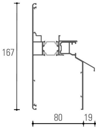
Figura 2.5e: Perfil 4805 + tapeta 4808.
