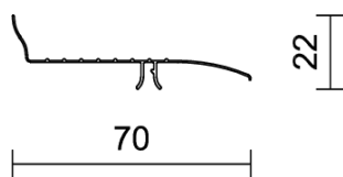
Figura 2.7: Vierendeaguas interno 1372.
