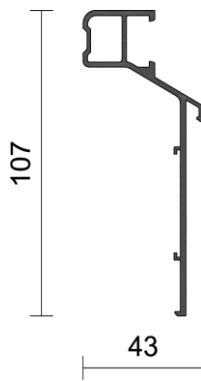
Figura 2.4e: Tapeta 4808 de aluminio recta con vierteaguas.
