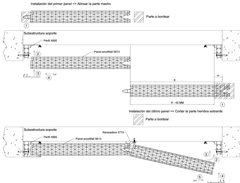
Figura 5.8: Instalación de los paneles inicial y final.
