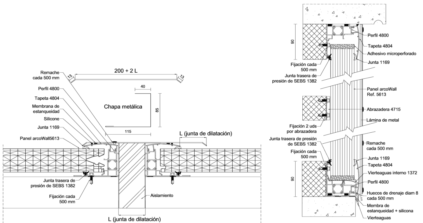
Figura 5.25: Junta de dilatación entre paneles con perfiles curvados.
